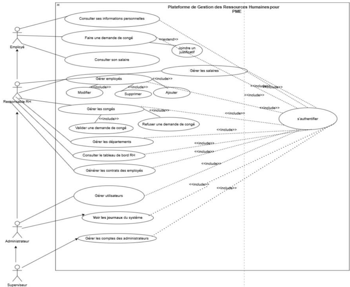
FIGURE 2.1 – Diagramme des cas d'utilisation
